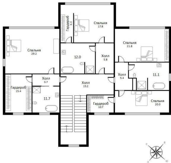
2 ЭТАЖ
