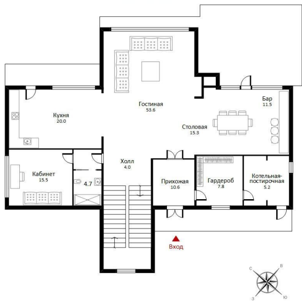
1 ЭТАЖ
